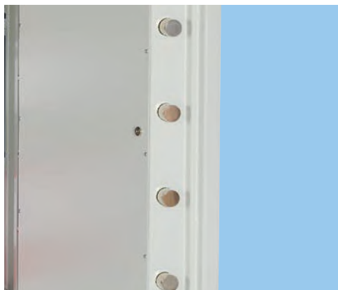
Dreiwandiger Türaufbau mit massiven Riegelbolzen
