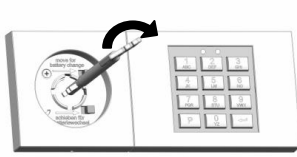
Abb. 5.5: Schlüssel im Uhrzeigersinn bis zum Anschlag drehen.
