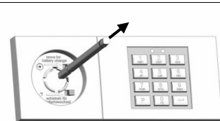
Abb. 5.3: Inbusschlüssel entfernen und Vierkantwelle herausziehen.
