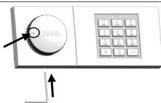
Abb. 5.1: Position Drehgriff (Markierung) merken. Inbusschlüssels in kleines Loch bis zum Anschlag eindrücken.
