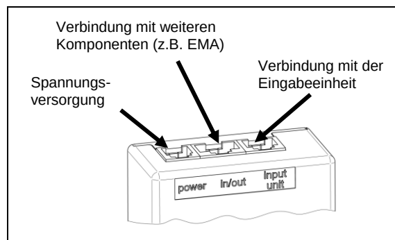
Abbildung 4: Anschlüsse am Schlossgehäuse
