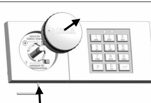
Abb. 5.2: Abziehen des Drehgriffes nach vorne, dabei Inbusschlüssel gedrückt halten.
